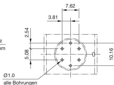
Bohrplan (Lötseite)
