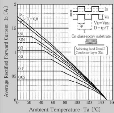
ディレーティングカーブ Ta-Io
