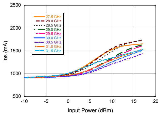
I_{DS} vs. P_{IN}
