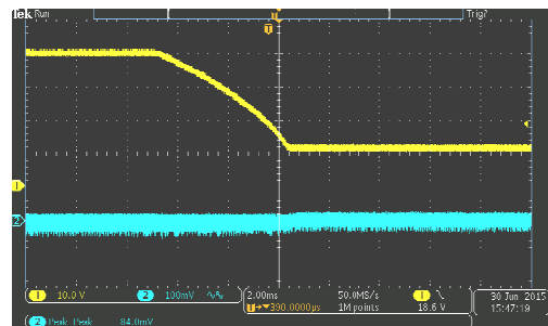
Vin=40V-12V
