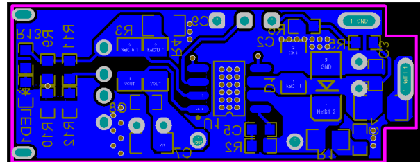
BOTTOM LAYER
