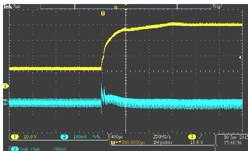
Vin=12V-40V
