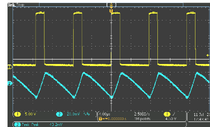
Vin=24V Vout=5V Iout=1A
