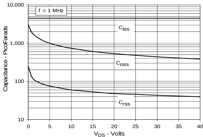
Fig. 11. Capacitance
