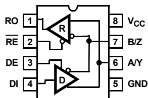
ISL83483, ISL83485 TOP VIEW
