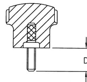
THREADED STUD
