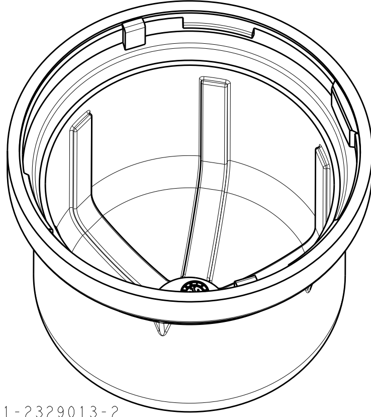
2329013-2 AND 1-2329013-2 SHOWN SCALE 2:1
