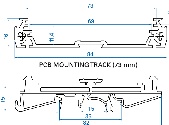
DIN RAIL MOUNTING FOOT (73mm)
