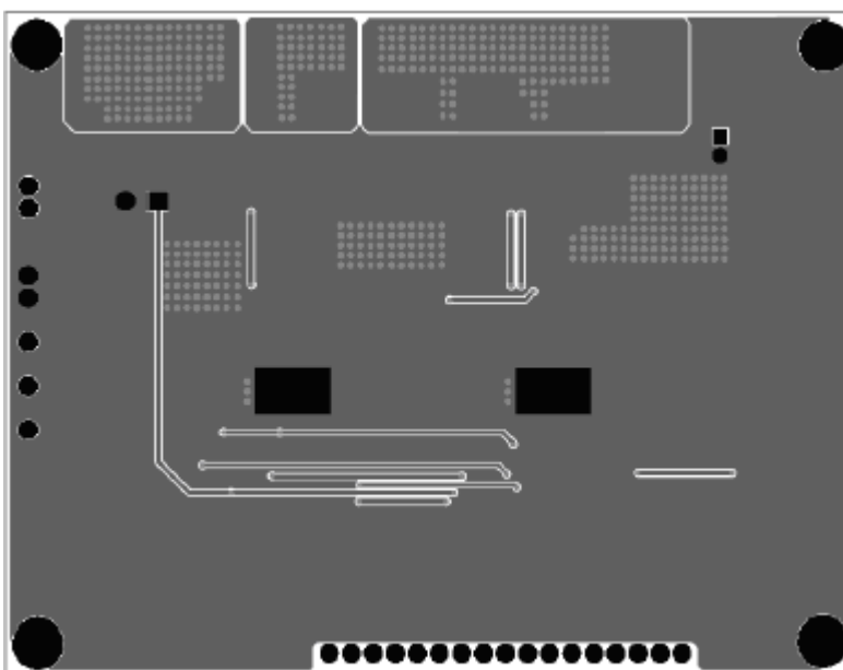
Figure 2—Bottom Layer
