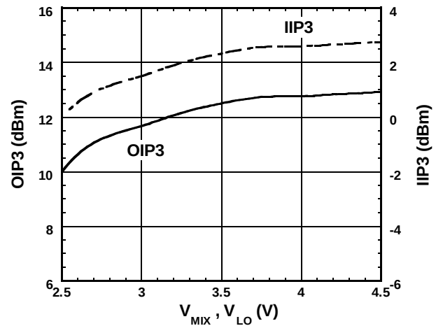
OIP3, IIP3 vs. V_{\text{MIX}}, V_{\text{LO}}
