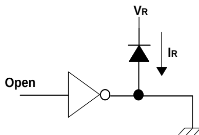
Fig. 7 IR Test Circuit
