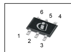
PG-SOT363
