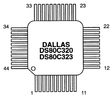
44-PIN TQFP
