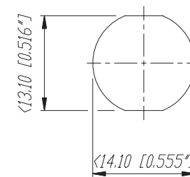
Frontplattenausschnitt (Rückseite) Panel cut out (rear side)
