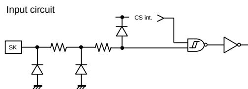
Figure 41. Input circuit (SK)
