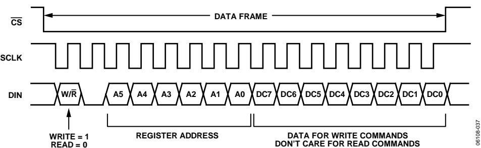
Figure 26. DIN Bit Sequence
