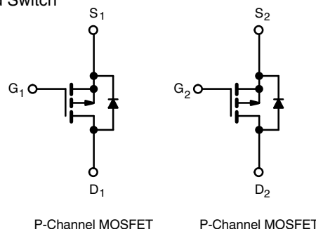
P-Channel MOSFET
