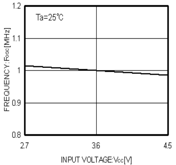
Fig.79 V CC -F osc
