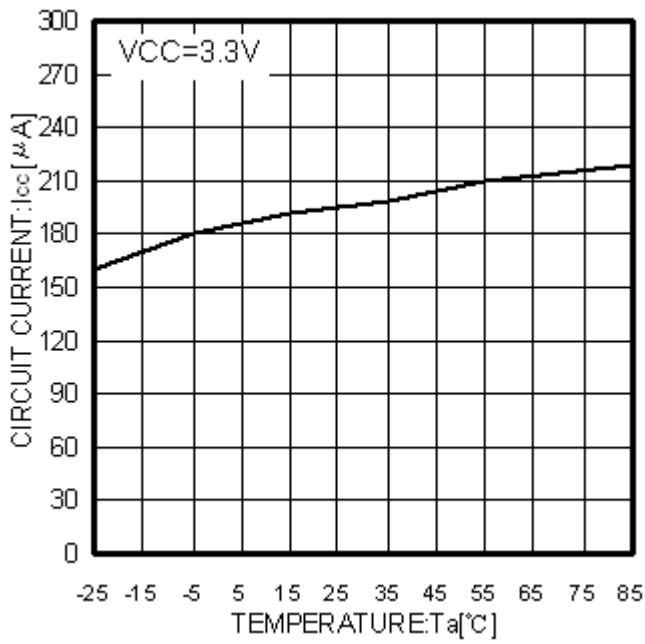
Fig.78 T a -I cc
