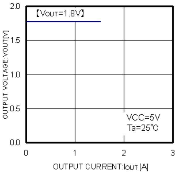
Fig.12 Iout-Vout
