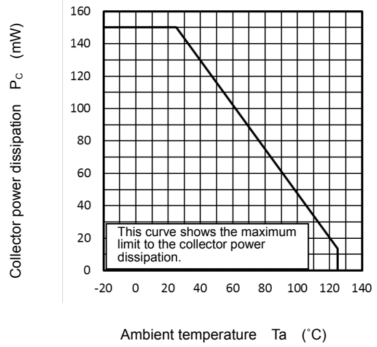
P_C - T_a
