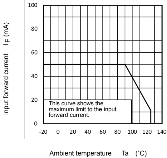
I_F - T_a
