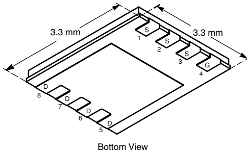
PowerPAK 1212-8
