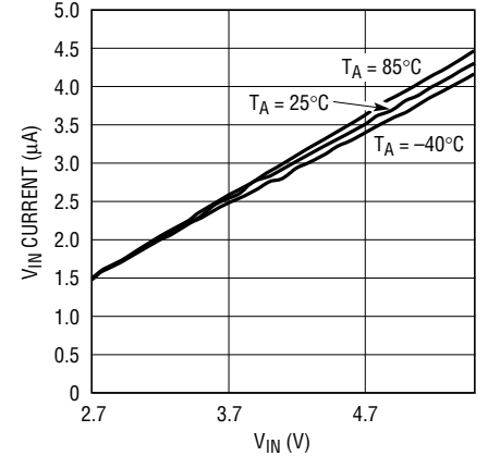
VIN Shutdown Current vs VIN Voltage
