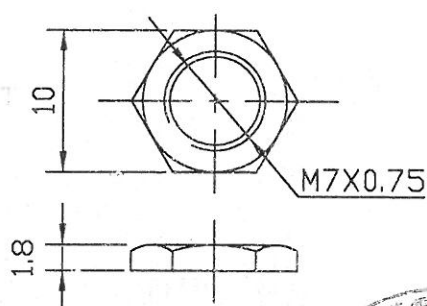
NUT 1 PC
