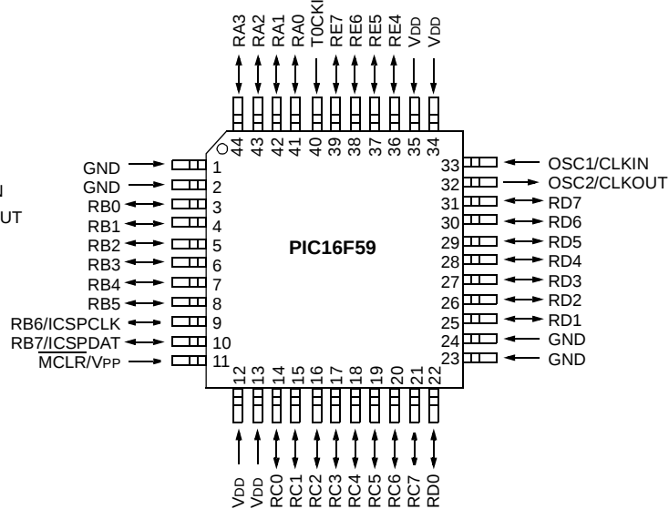
TQFP
