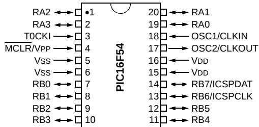
SSOP
