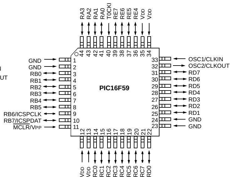
TQFP
