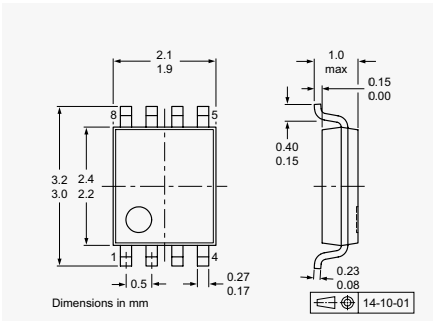
SOT765-1 DC
