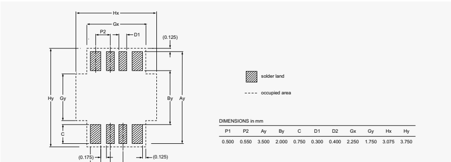
SOT765-1 DC
