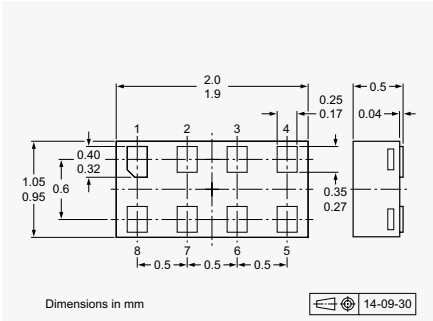
SOT833-1 GT
