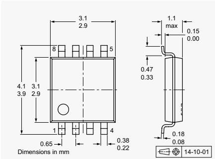
SOT505-2 DP
