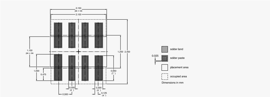
SOT833-1 GT
