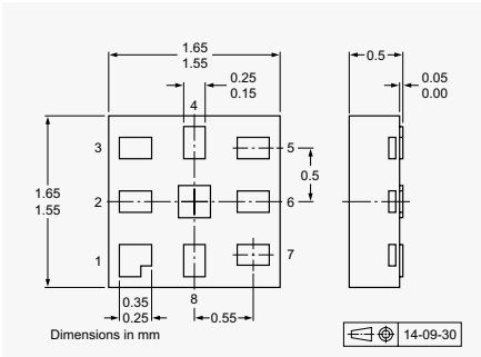
SOT902-2 GM
