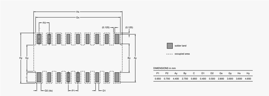
SOT505-2 DP
