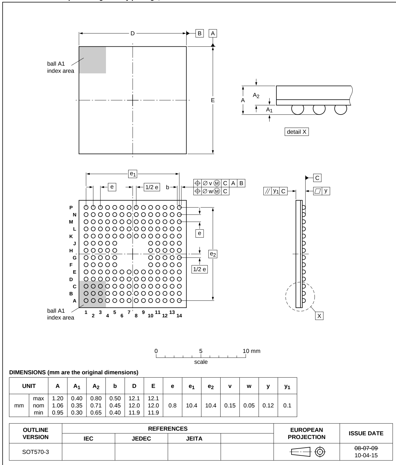
SOT570-3
