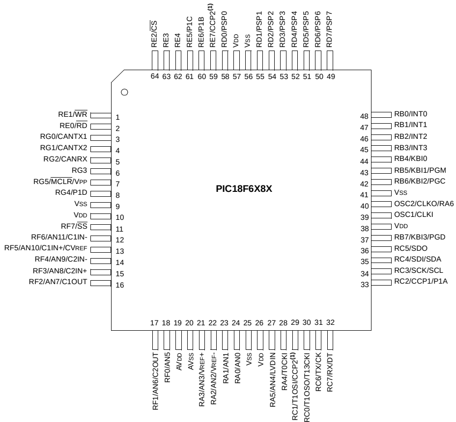
64-Pin TQFP
