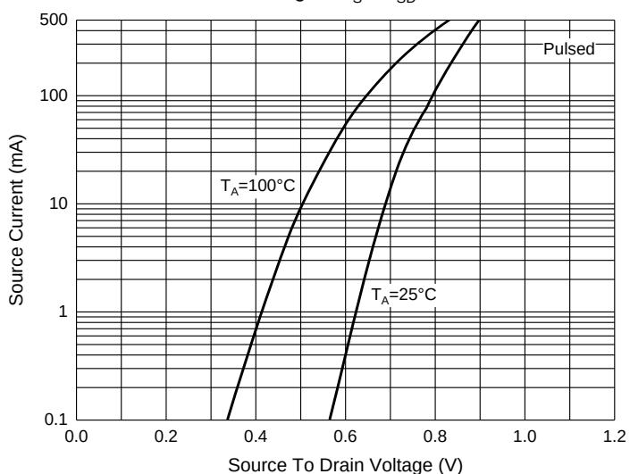
Fig. 5 - I_S - V_{SD}
