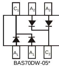
BAS70DW-05*
