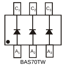
BAS70TW
