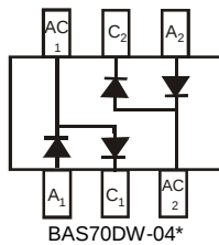
BAS70DW-04*
