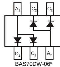
BAS70DW-06*
