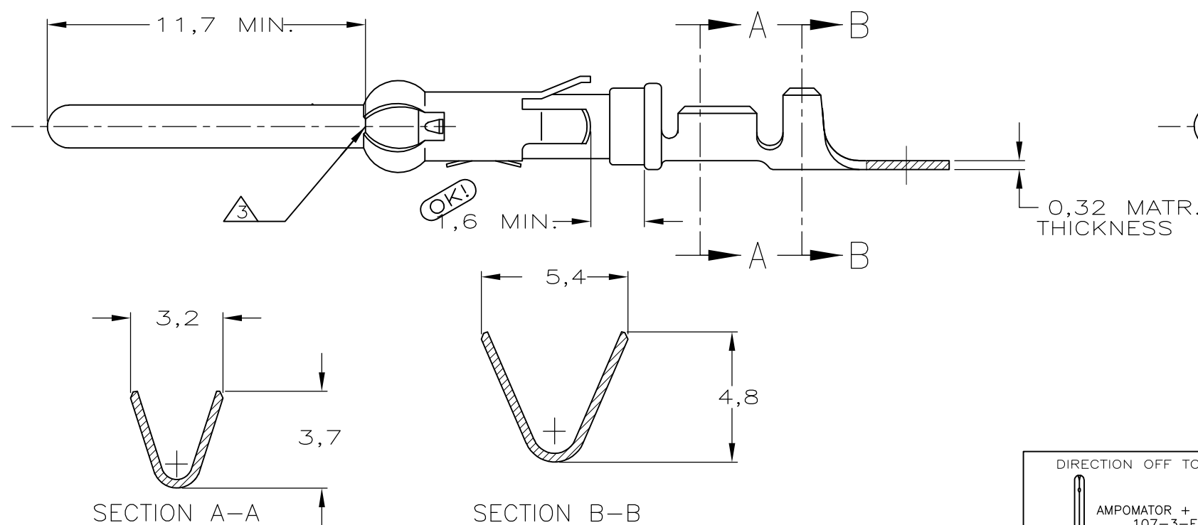
SECTION A-A
