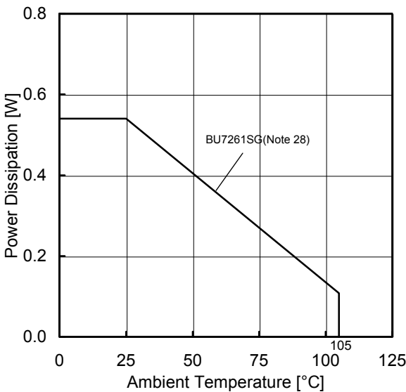
(d)BU7261SG
