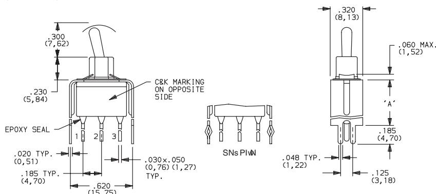
E101MD1__BE SPDT
