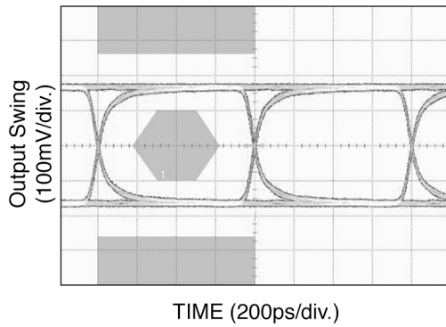
1.25Gbps Data
