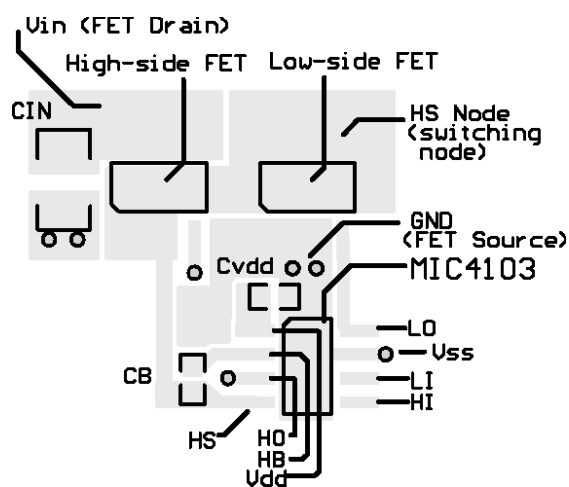
Top Side
