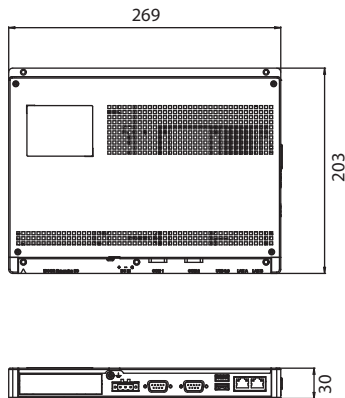
TPC-B200
