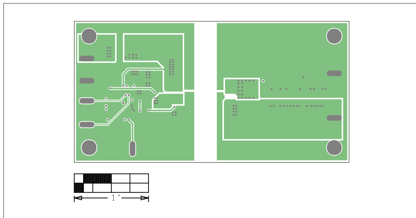
INNERLAYER3
