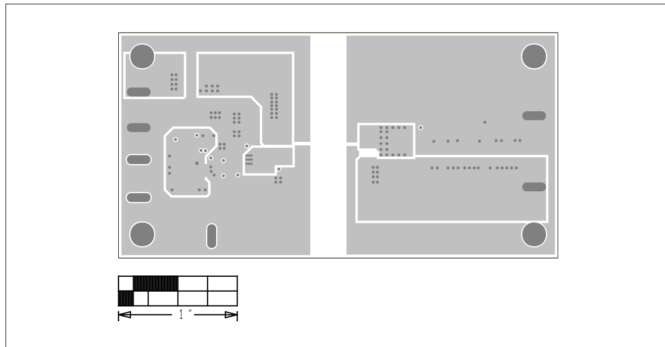
INNERLAYER2
