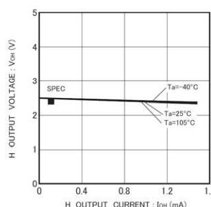
Fig.36 H output voltage V_{OH} - I_{OH} ( V_{CC}=2.5V )
