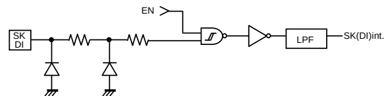
Fig.39 Input circuit (SK, DI)
