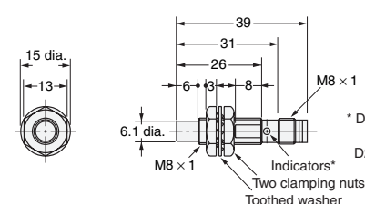
Diagram 29 E2E-X4MD□-M3G/E2E-X2ME□-M3/X2MF□-M3
