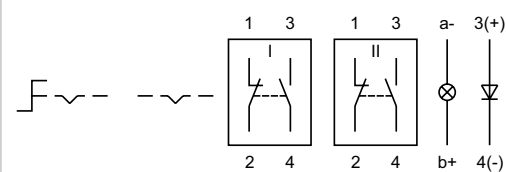
Wiring diagram 24
