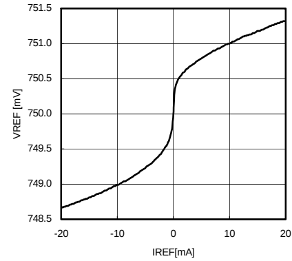
Fig.7 IREF-VREF (DDR3)
