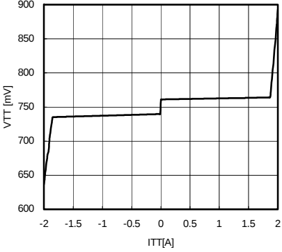
Fig.6 ITT-VTT (DDR3)
