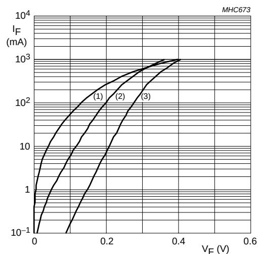
PMEG2010BEA/PMEG2010BEV
