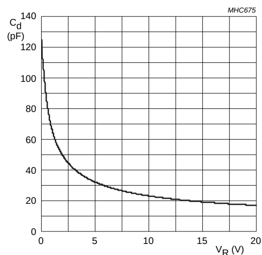
PMEG2010BEA/PMEG2010BEV
