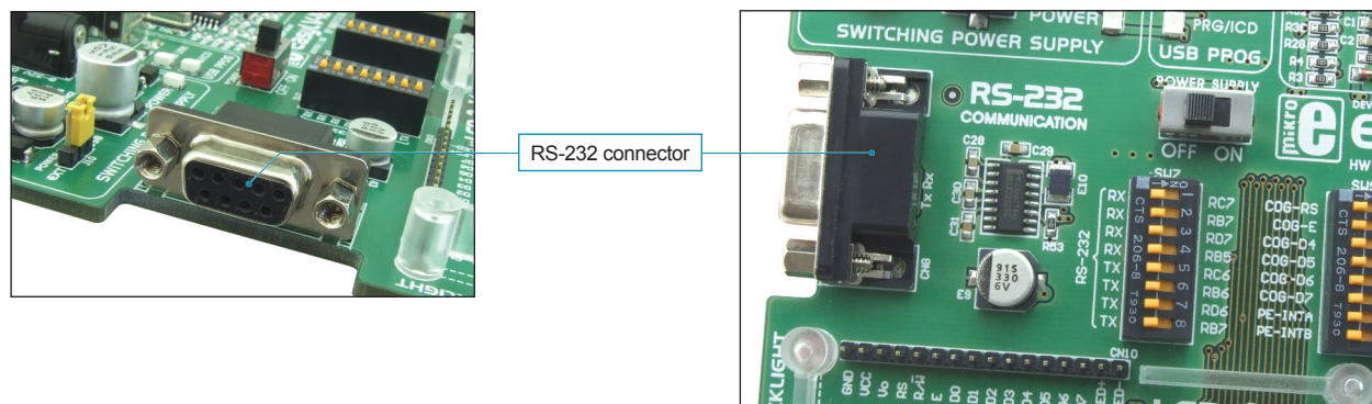
Figure 11-1: RS-232 module
