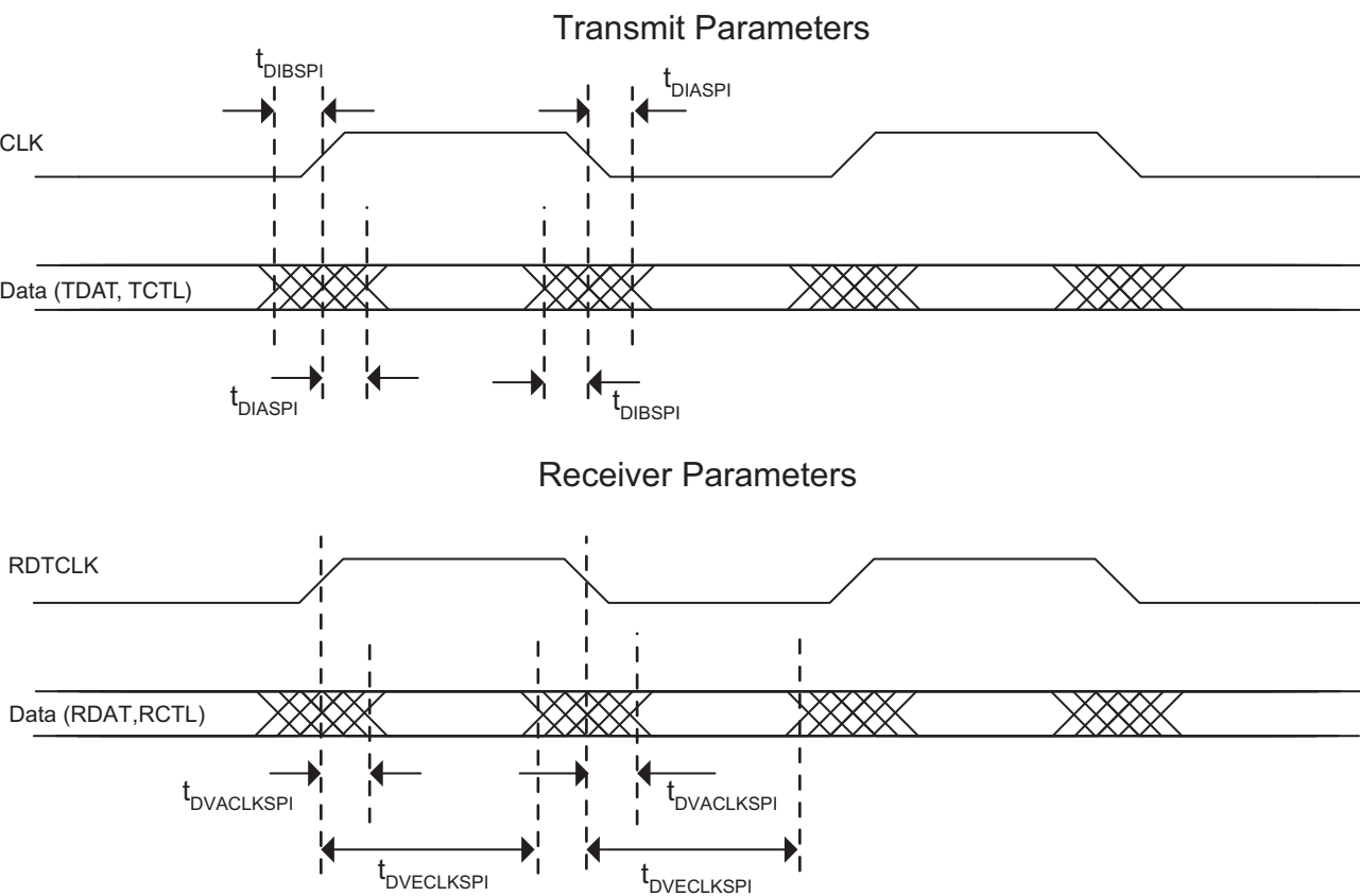
Figure 3-6. SPI4.2 Parameters
