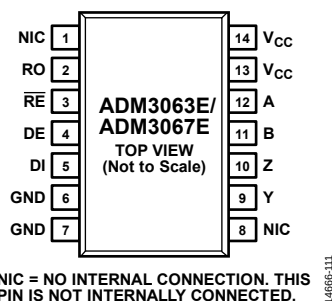
Figure 13. ADM3063E/ADM3067E 14-Lead SOIC_N Pin Configuration
