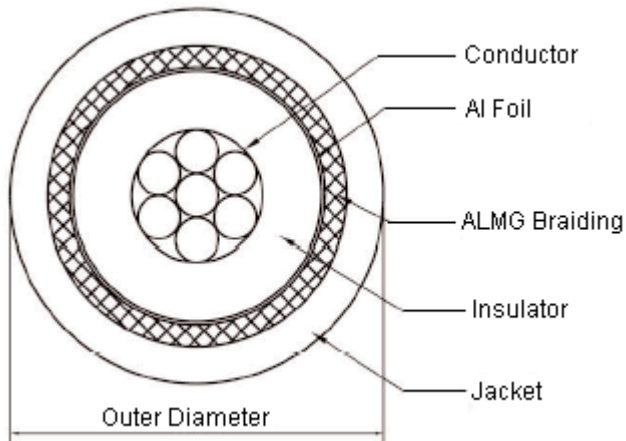
Dimensions : Millimetres
