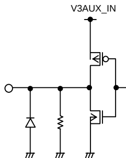
8pin&lt;PERST#&gt;
