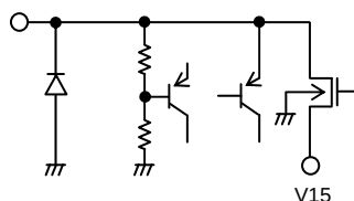
11,13pin&lt;V15&gt;
