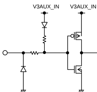
10pin&lt;CPPE#&gt;
