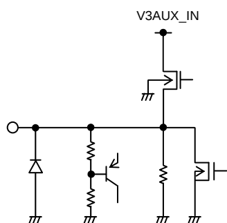
15pin&lt;V3AUX&gt;
