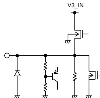
3,5pin&lt;V3&gt;
