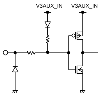
10pin&lt;CPPE#&gt;
