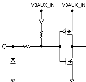
1pin&lt;SYSR&gt;
